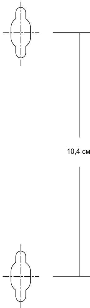
PC23 Шаблон настенной установки
